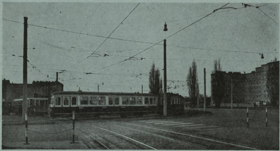
Fahrleitungsanlage nach System Kummler & Matter, ausgeführt für die Wiener Stadtwerke-Verkehrsbetriebe
