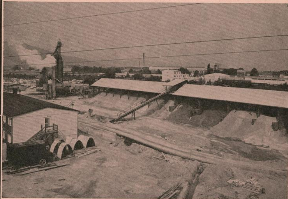
Ansicht des Asphaltmischwerkes Wien-Nord, Strebersdorf
