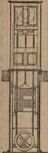
Speisen-Aufzug für Handbetrieb.
