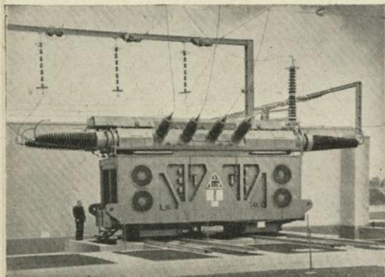
Drehstrom-Transformator 100.000 kVA, 220.000/110.000 V, für Umspannwerk Bisamberg bei Wien. Hersteller ELIN AG. Wien, Werk Weiz
