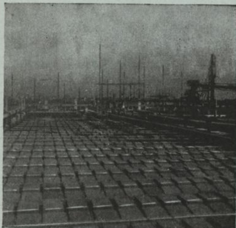
Bau der Wohnhausanlage WIEN XX, Kapaunplatz Verlegte Ebenseer Hohlsteindecke vor dem Verguß
