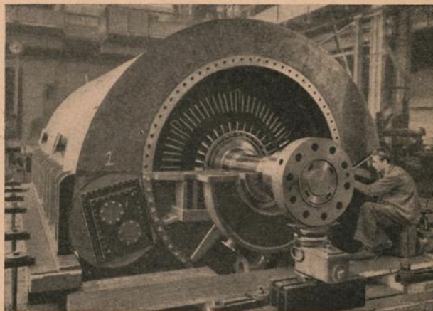
Turbogenerator 80.000 kVA, 3000 U/min. (mit Wasserstoffkühlung) - DKW-Simmering
