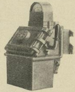
Gußgekapselter Motorschutz PHYLAX Gg
