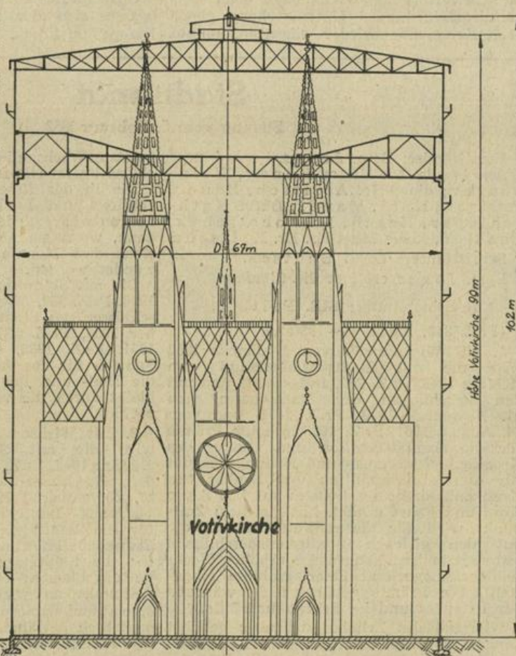
Wasserloser Gasbehälter 300.000 m 3 : Gaswerk Wien-Leopoldau
