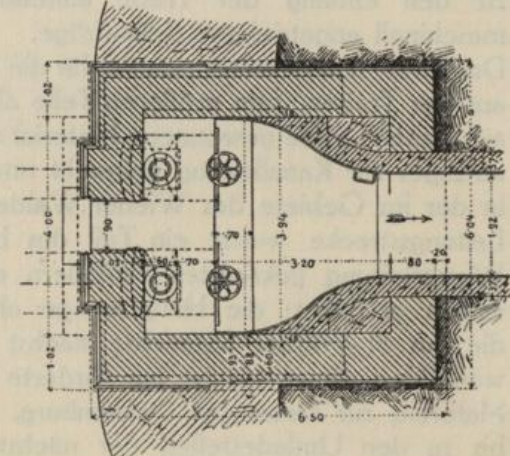
Grundriß.
