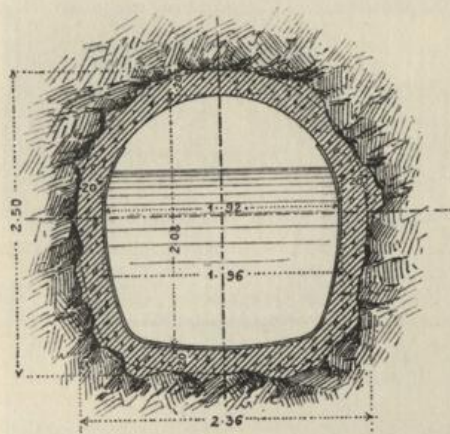
Stollenprofile für das Gefälle 0-22 ‰/100.
