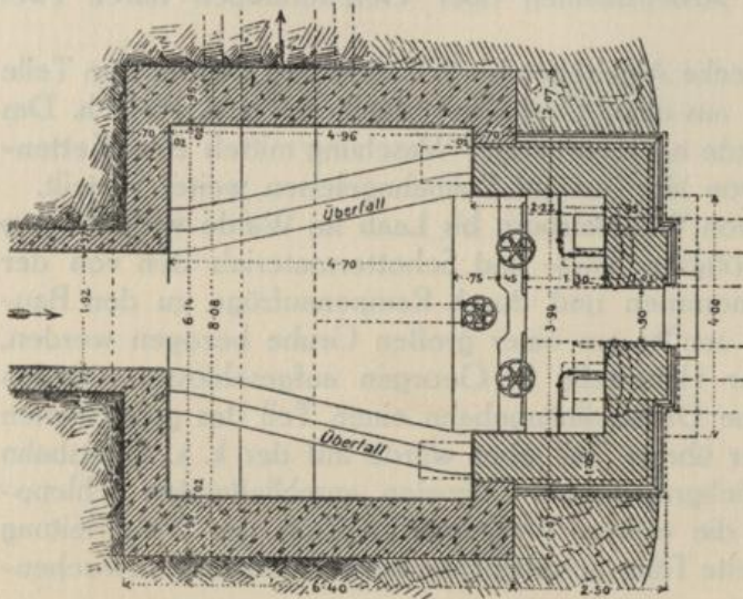
Grundriß.
