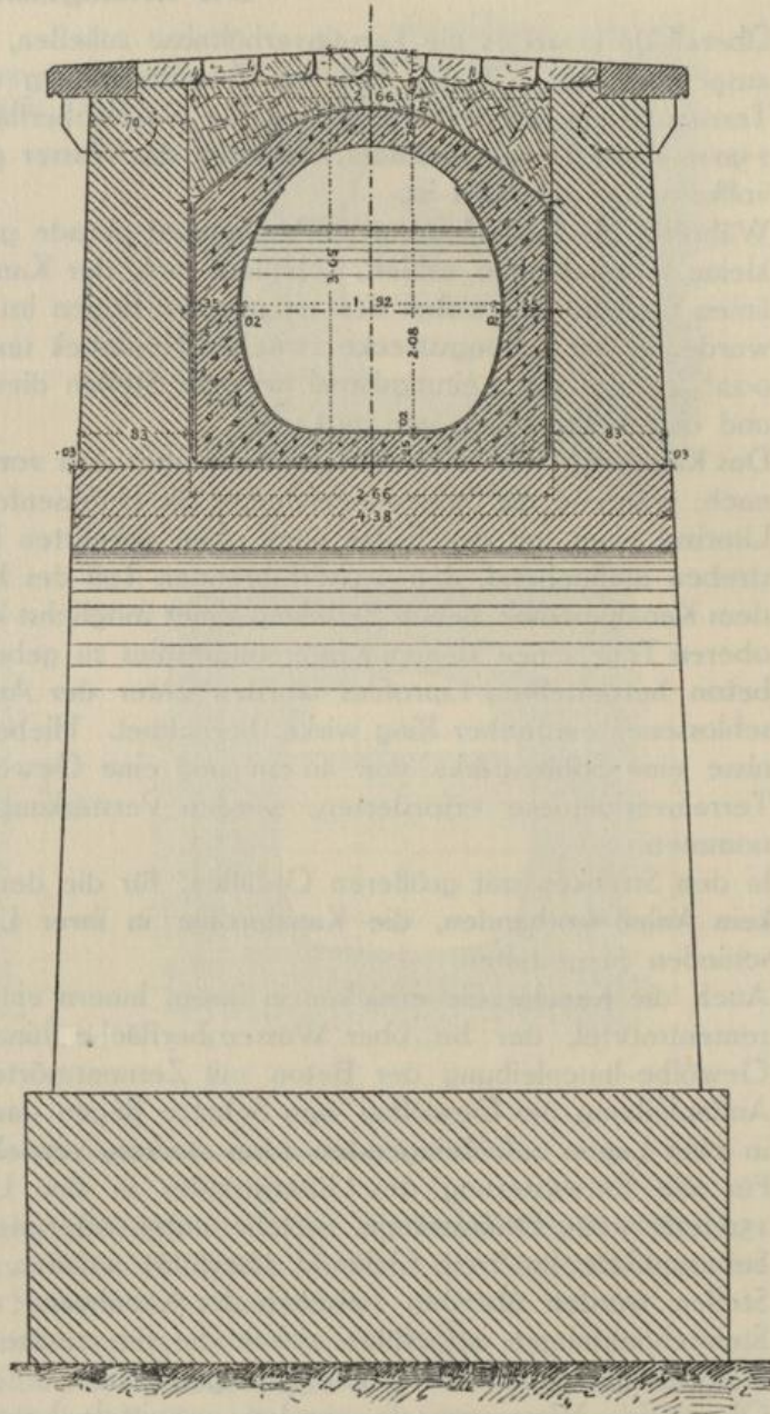
Aquäduktprofil für das Gefälle 0.22‰.
