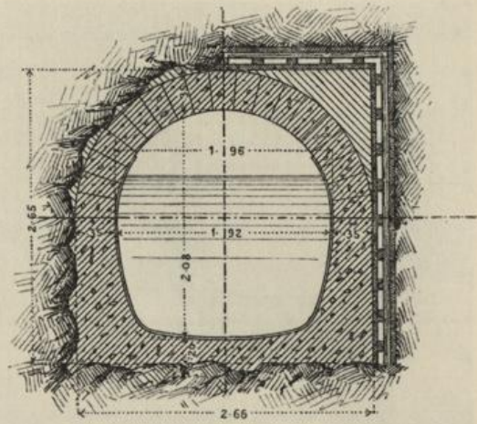
Stollenprofile für das Gefälle 0-22 ‰/100.
