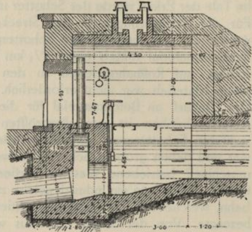
Siphonauslaufkammer. Längenschnitt.
