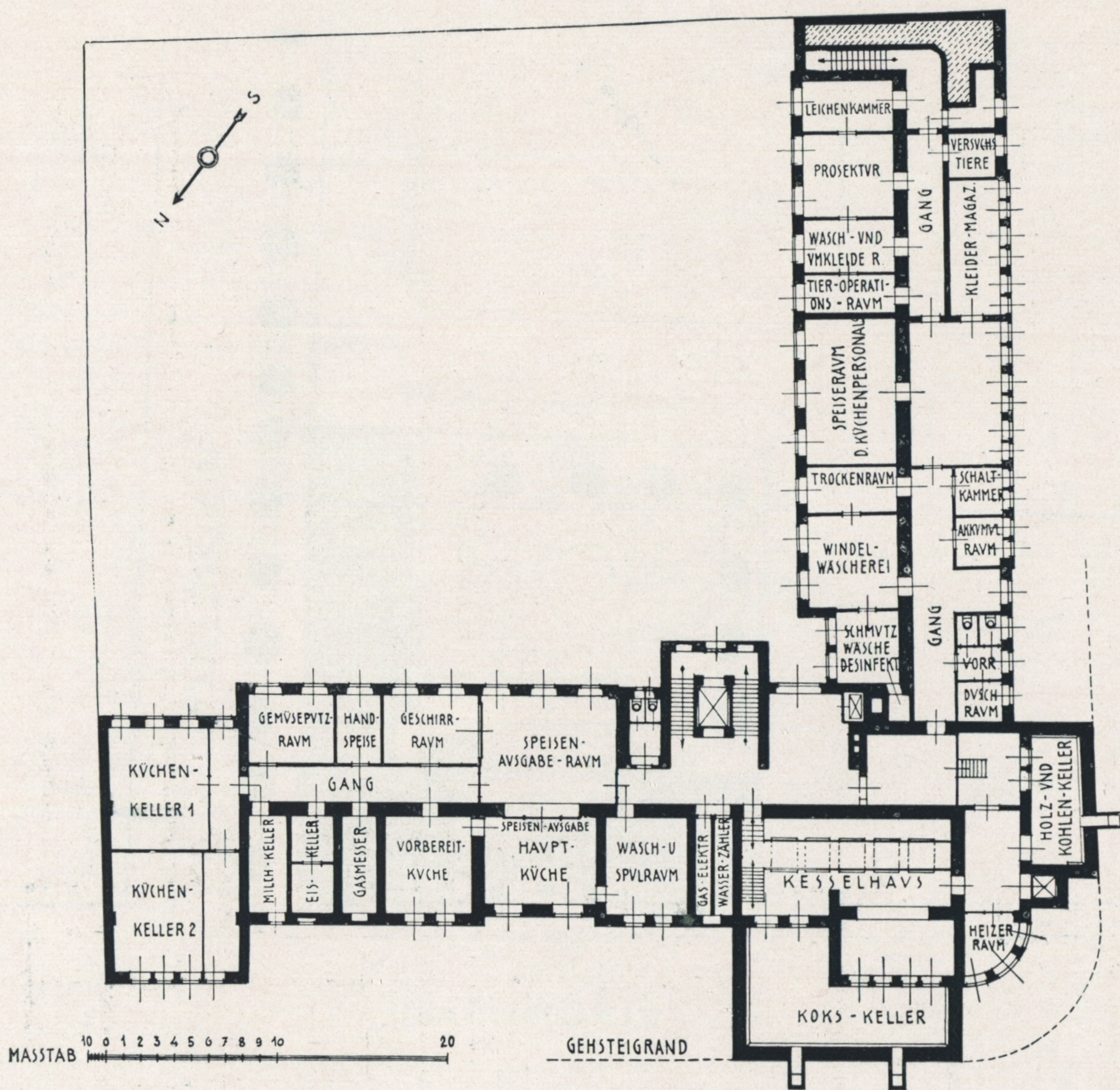
Kellergeschoß.
