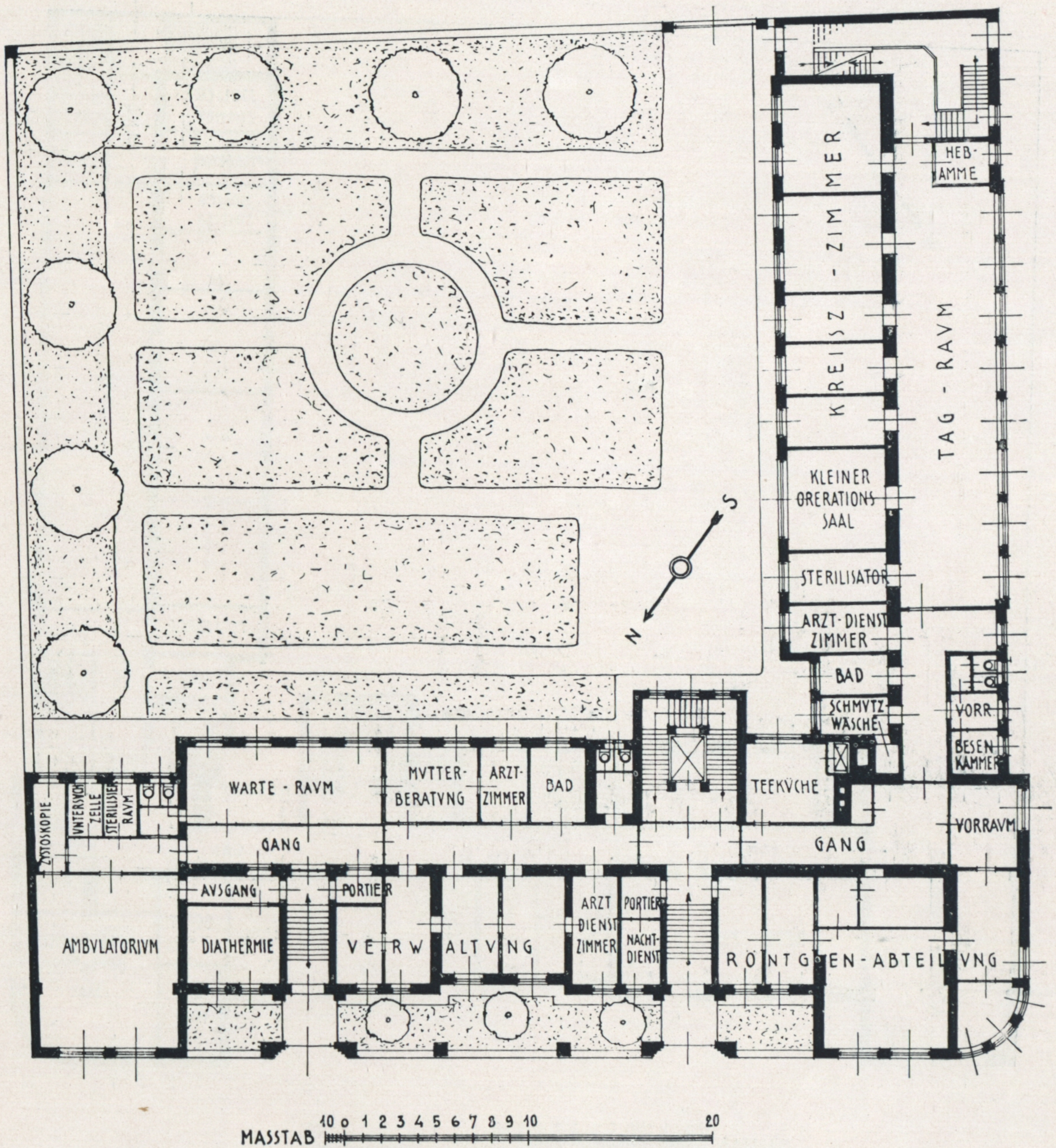
Erdgeschoß.
