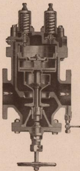
Dampfgesteuertes Druckminderventil
