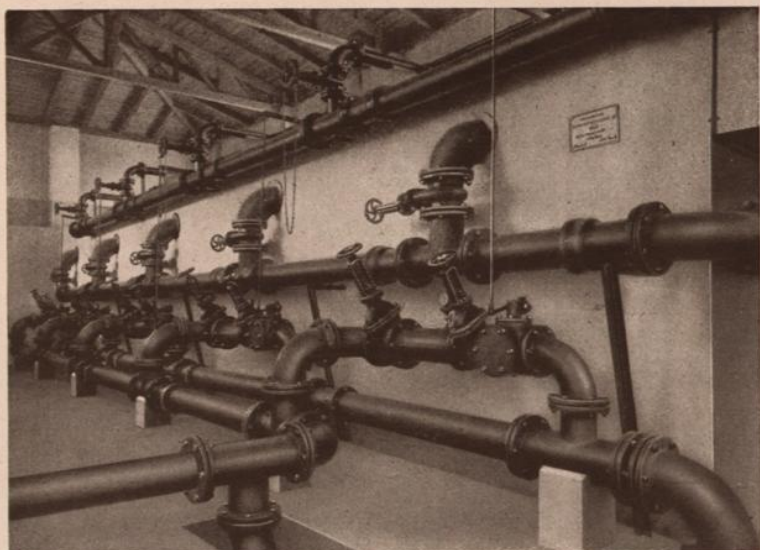
Filtrations- und Entkeimungs-Anlage des Bades der Gemeinde Wien am Kongreßplatz (Teilansicht)
