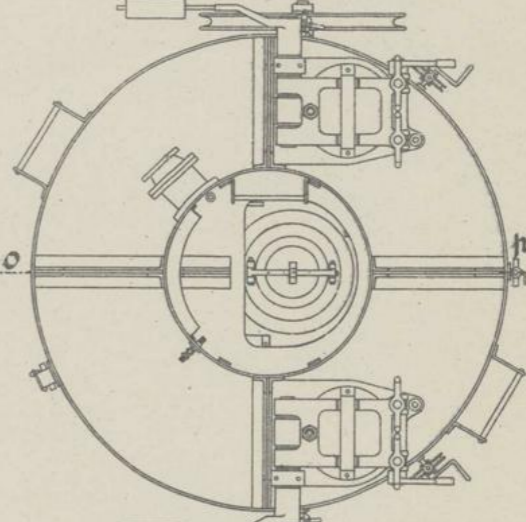
Fig. 8. Untere Ansicht.
