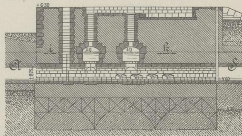
Schnitt e,f in der Richtung des Umlaufcanales.
