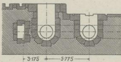
Horizontalschnitt i,k.
