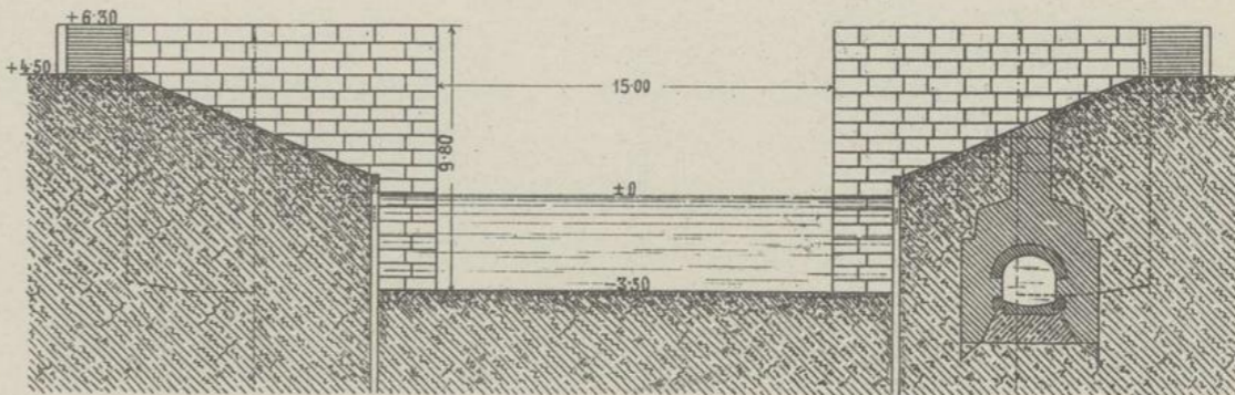
Stirn-Ansicht des Einlaufs.
