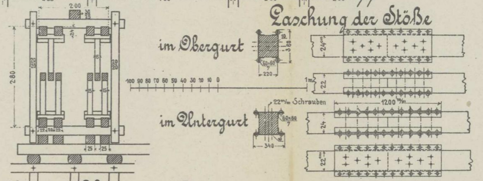
Querschnitt des Kow'schen Trägers.
