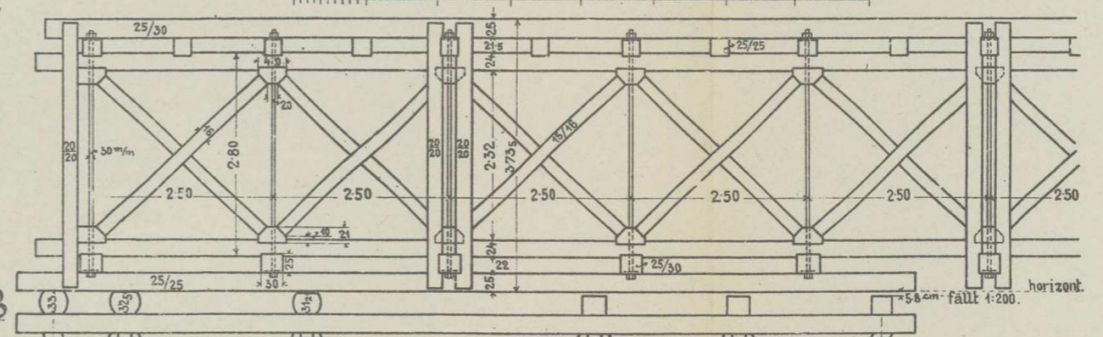
Detail des Kowischen Trägers u. der Auflagerung.
