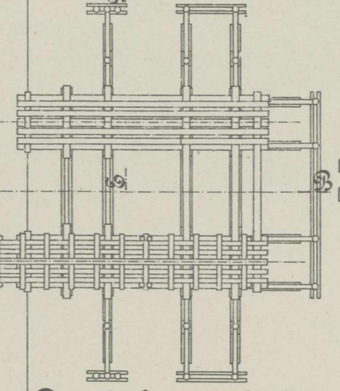
Draufsicht nach abgehobenem Träger.
