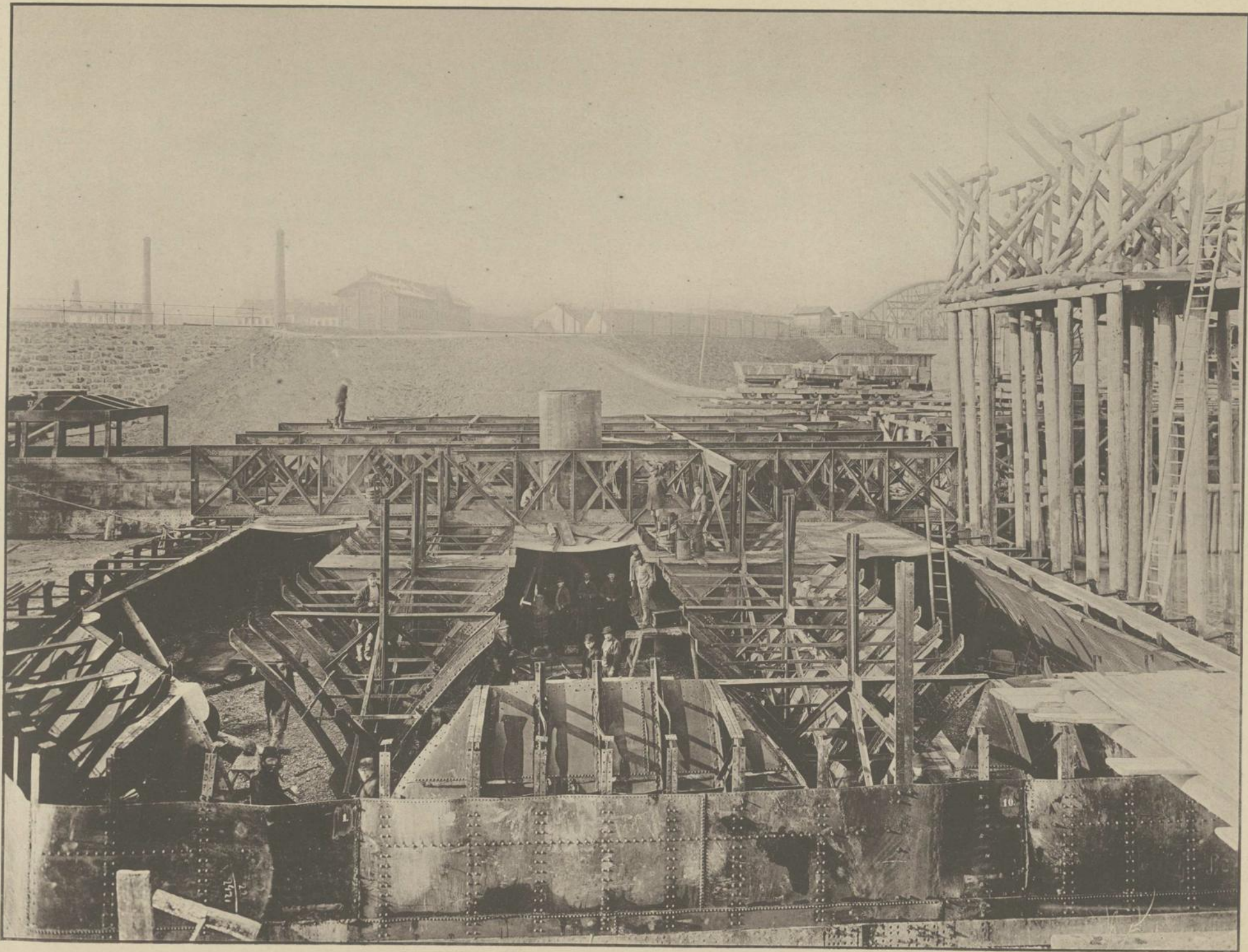
Der Caisson für das Unterhaupt der Kammer Schleuse in Montierung auf der Sohle der Baugrube. — Die Schneide befindet sich im Niveau des Nullwassers. — Wasserstand: 1.45 m unter Null.
