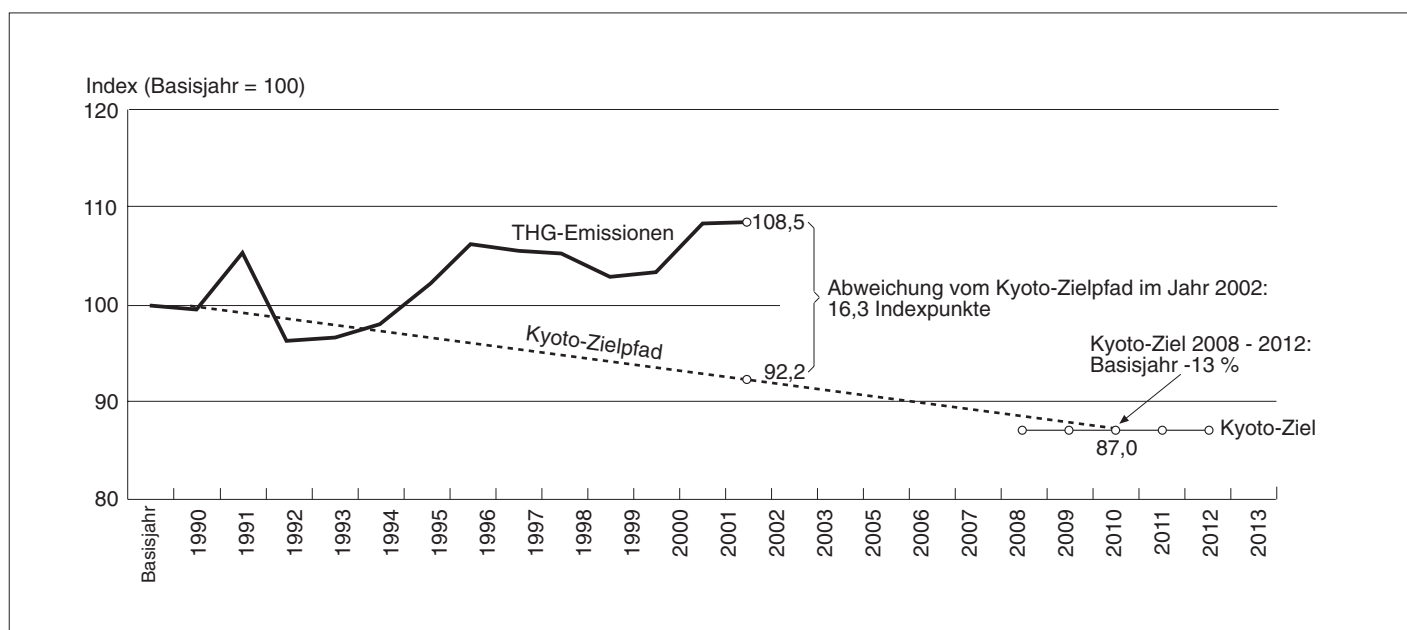
Abb. 14: Treibhausgas-Emissionstrend 1990 - 2012
