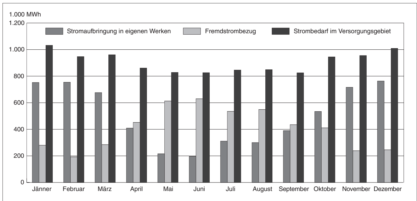
Abb. 23: Wienstrom - Stromaufbringung und -verteilung 2003
