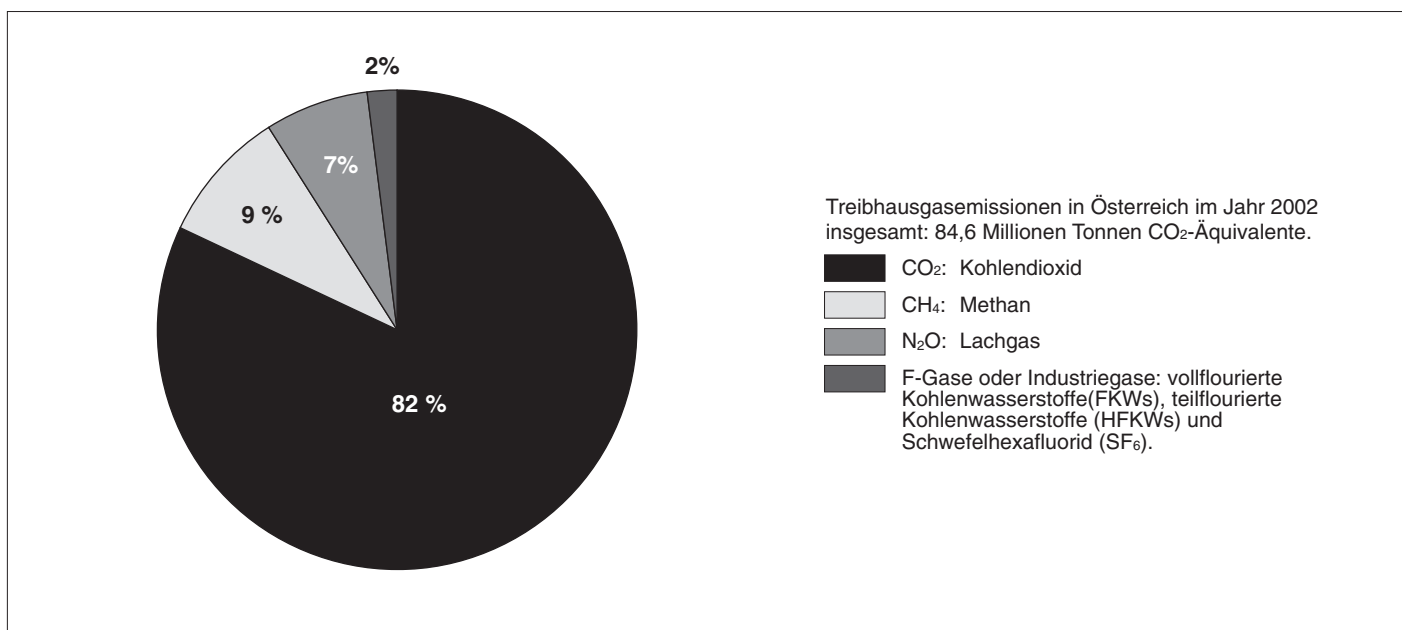
Abb. 13: Emissionen von Treibhausgasen in Österreich 2002
