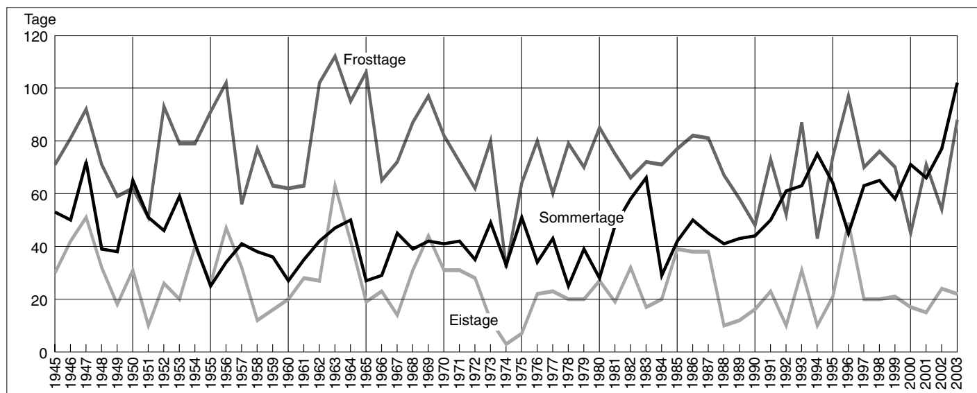
Abb. 5: Sommer-, Frost- und Eistage 1945 - 2003
