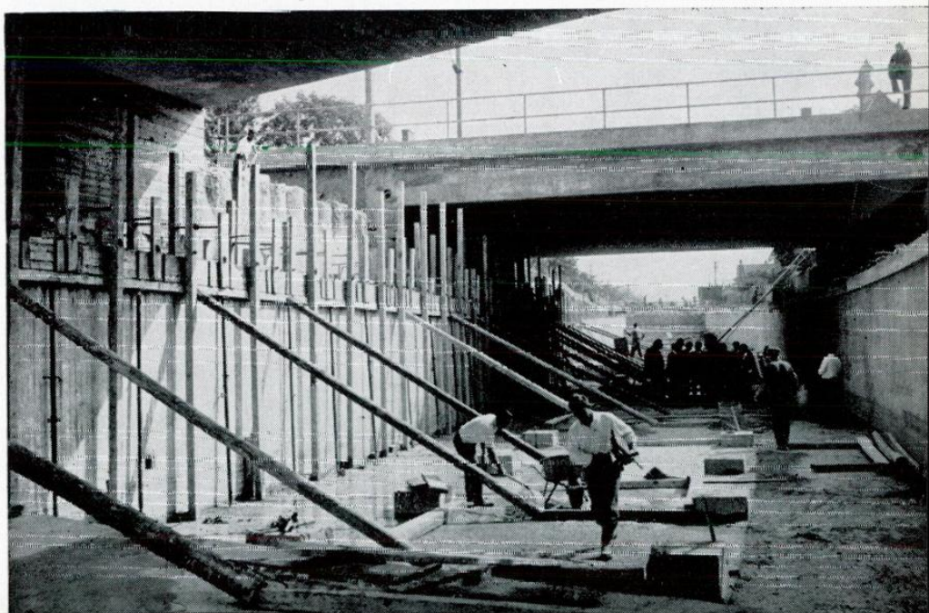
Die Baustelle der Unterführung der Südbahntrasse durch die Ketzergasse in Liesing
