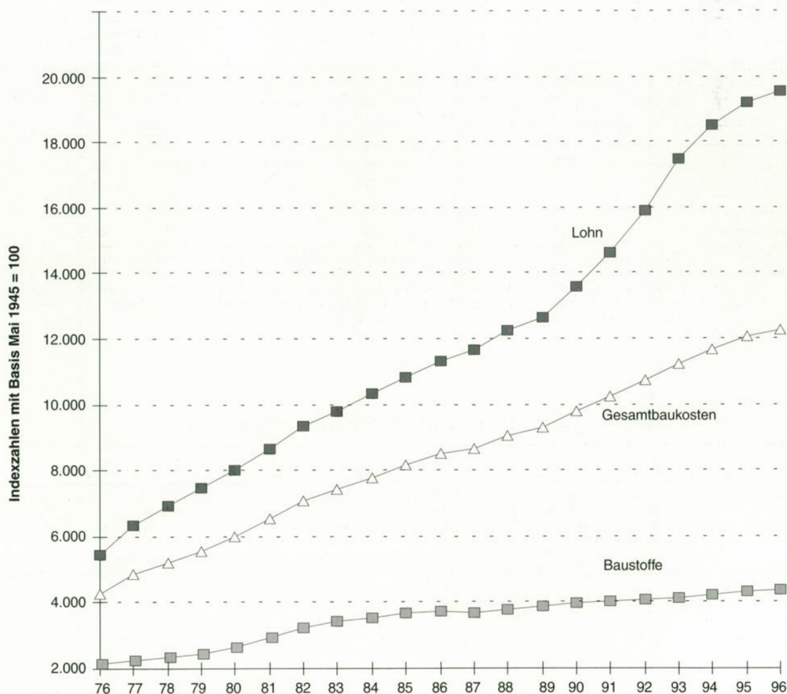
Entwicklung des Baukostenindex für den Wohnungsbau 1976 – 1996
