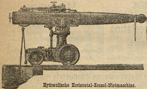
Hydraulische Horizontal-Kessel-Nietmaschine.
