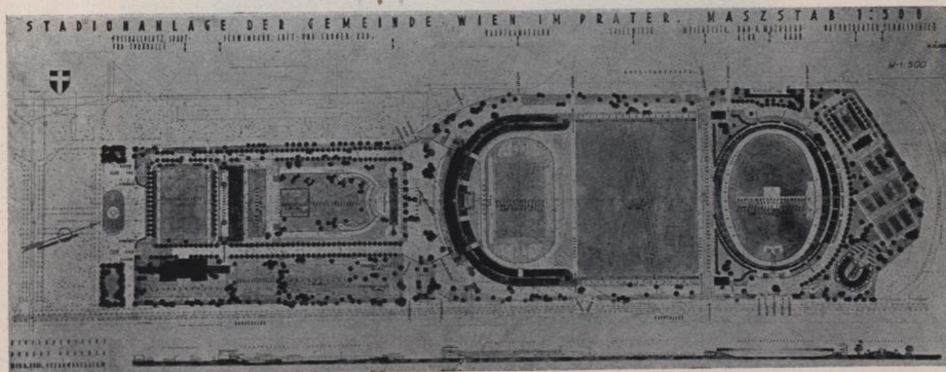
STUDIE ZUR WIENER STADION-ANLAGE 1927
