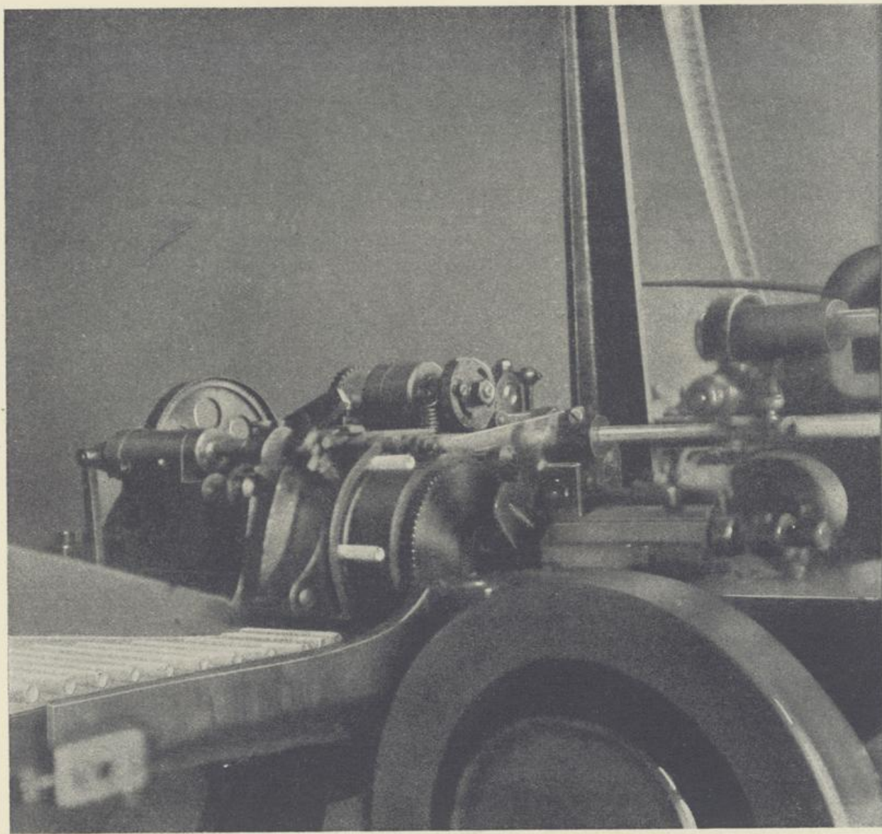
Teil einer Hülsenmaschine
