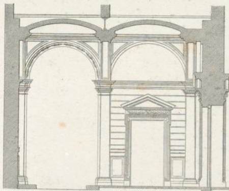
SCHNITT (COUPE) D-C
