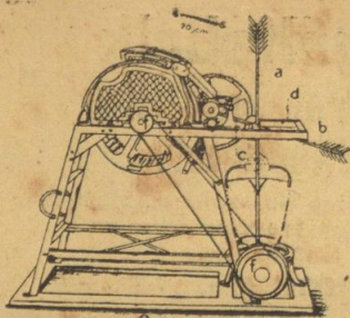
Aufdrehsapparat f. Handbetrieb. Aufdrehsapparat f. Kraftbetrieb
