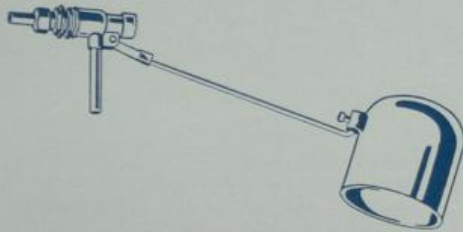
S. 7641 Messing-Schwimmerhahn \frac{3}{8} " mit Rauschröhr- chen und Kupfer-Schwimmglocke. S. 7641a. Mit Regulierung, sonst wie S. 7641.
