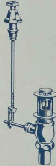
S. 8136 Ab- und Überlaufvorrichtung mit Umlegehebel für Waschtische, mit kombiniertem Ab- und Überlauf, mit außen- liegendem Gestänge und Ab- und Überlaufventil 1/4"
