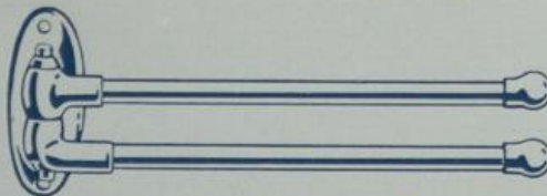
S. 7861 einteilig, S. 7862 zweiteilig. 24 mm stark, 550 mm lang, gekröpft.
