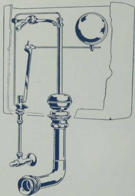
S. 7654 Komplette Absauge-Innengarnitur, Spezialmodell für Steingut-Rücken- reservoir mit Bodenventil, Spülrohr- bogen mit Verschraubung, Sauger mit Schwimmkugel und Druckhebel, Schwimmventil \frac{1}{2} " mit Schwimm- kugel, Eckregulierhahn \frac{1}{2} ", mit Guß- rosette und 2 Spülkastenstützen
