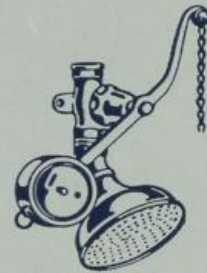
S. 7405 1/2" Zugdusche, bestehend aus: Kugelfallhahn mit Hebel, Gewicht, 1.50 m Messing- kette, Bogen und Brause- kopf
