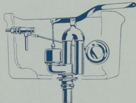
S. 7642 Komplette Innengarnitur für Steingut-Spül- kasten, bestehend aus: Messingsauger mit Holländerstutzen 32 mm \emptyset , Bleigewicht mit Kette, Messinghebel und Messing-Schwim- merhahn S. 7640. Alle sichtbaren Teile vernickelt oder nickel- verchromt.
