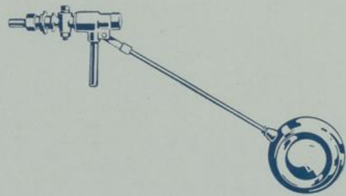
S. 7640a Messing-Schwimmerhahn \frac{3}{8} " mit Regulierung, sonst wie S. 7640
