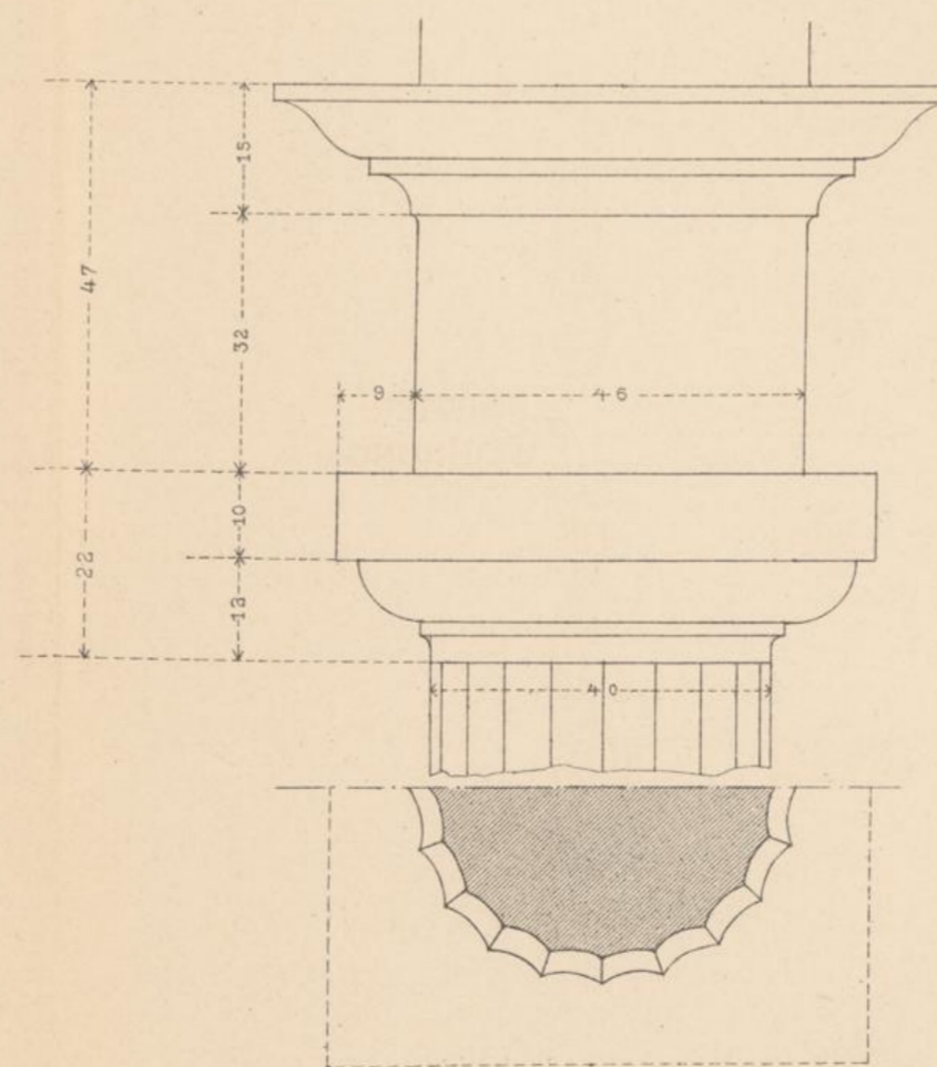
ARCHITRAV UND KAPITÄL.
