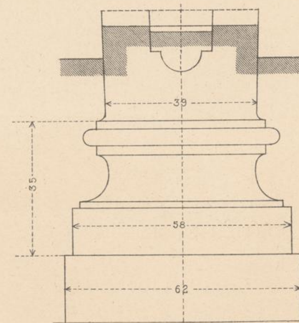
KÄMPFER BEI DER NICHE.
