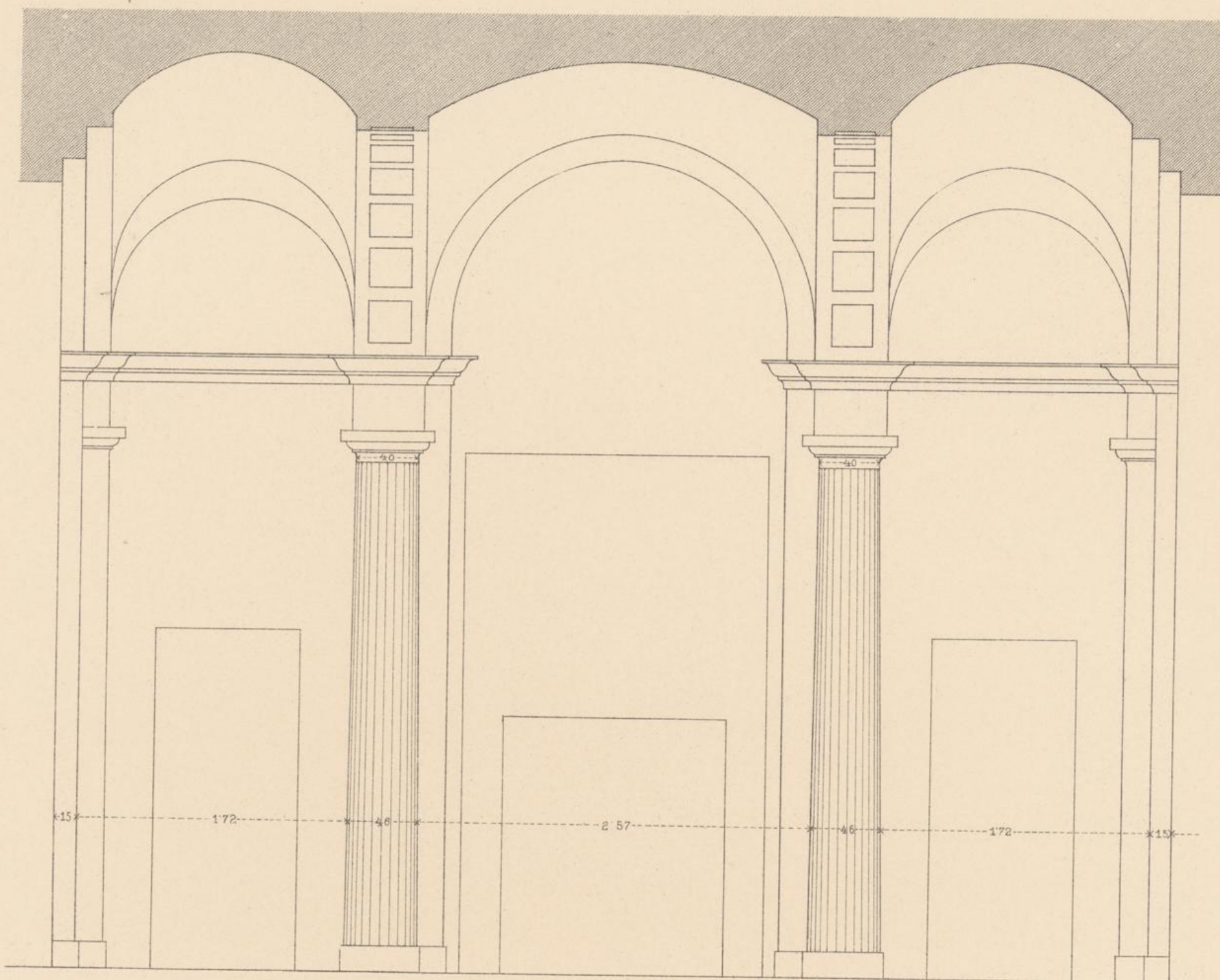
QUERSCHNITT NACH A. B.
