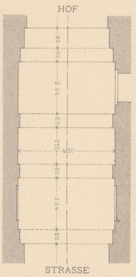
GRUNDRISS DES VESTIBULS IM HAUSE I, HERRENGASSE 10
