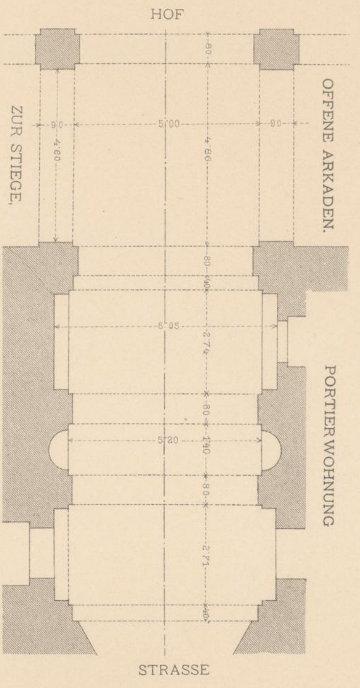
GRUNDRISS DES VESTIBULS IM HAUSE I, HERRENGASSE 8.
