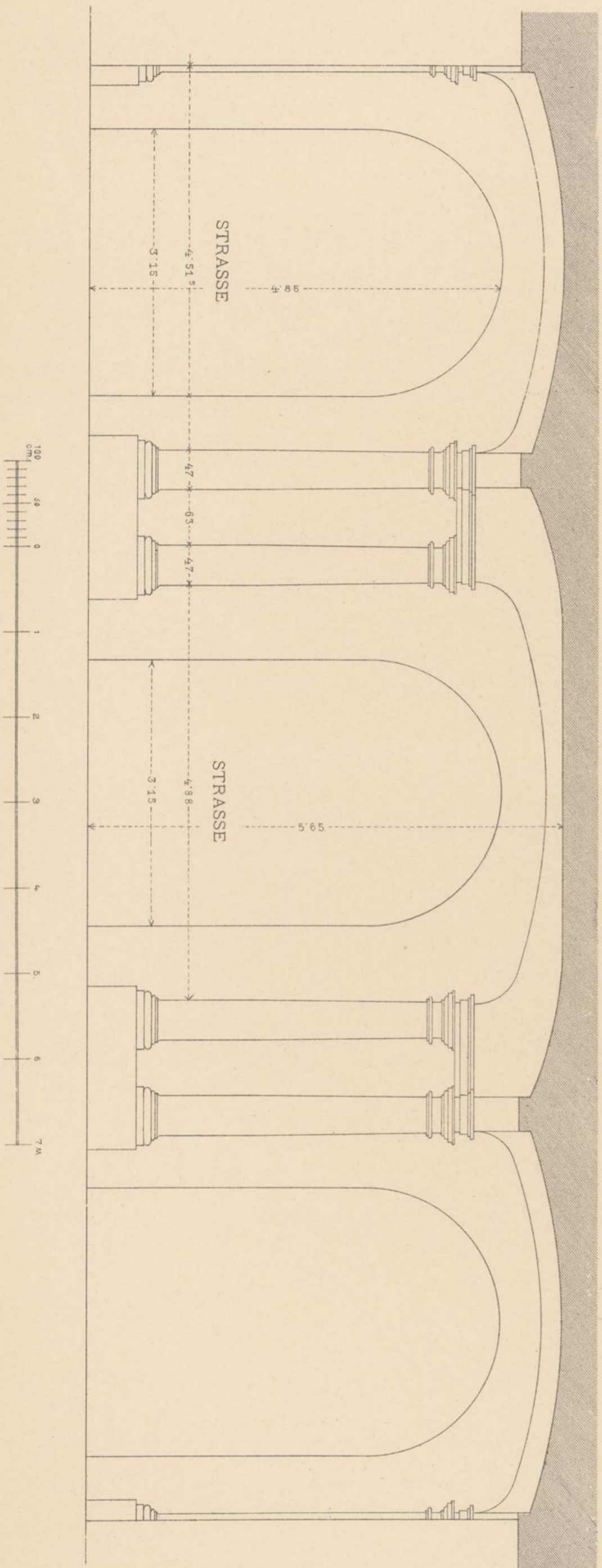
QUERSCHNITT NACH C. D.
