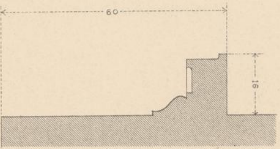
ARCHITRAV UND KÄMPFER ÜBER DEN 3/4 SÄULEN.
