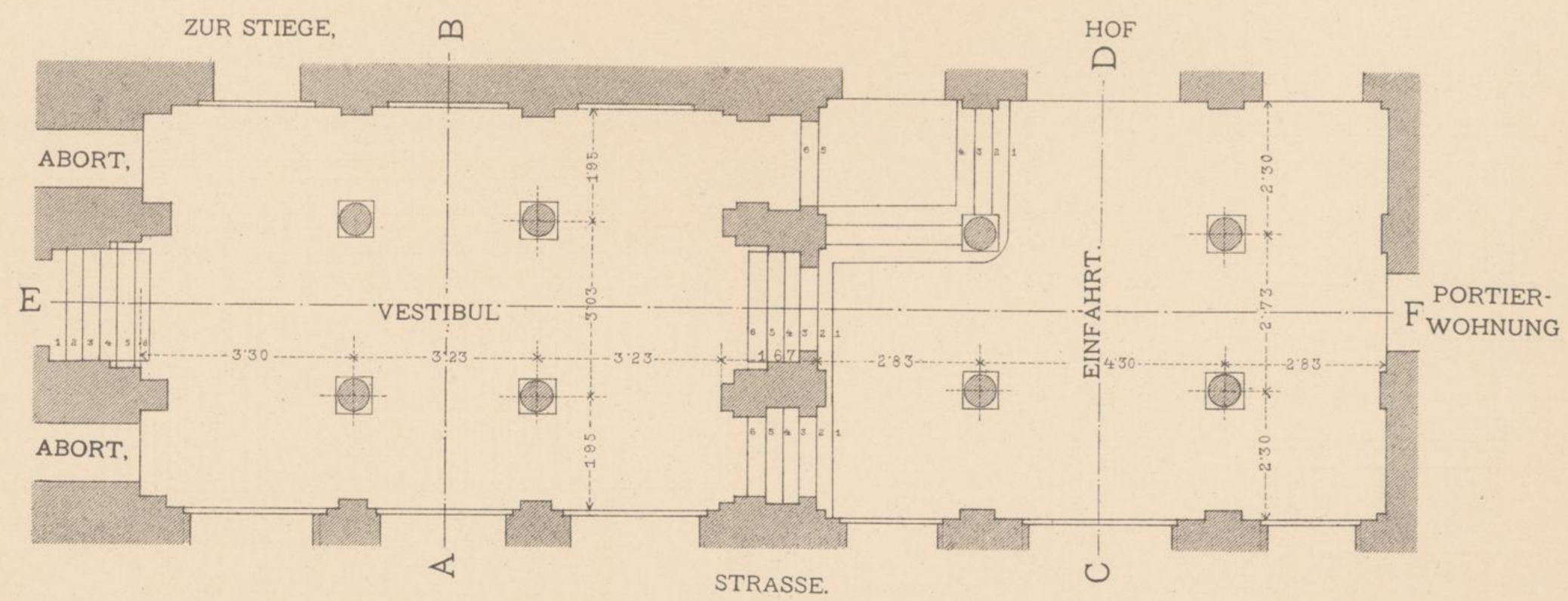
GRUNDRISS
