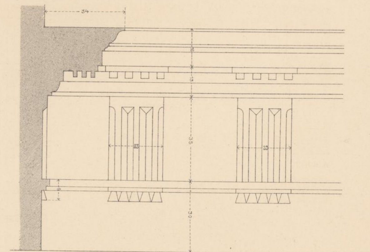
GESIMS IN DER EINFÄHRT.
