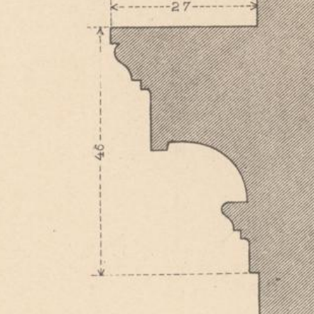
DETAIL DES GROSSEN KÄMPFERS.
