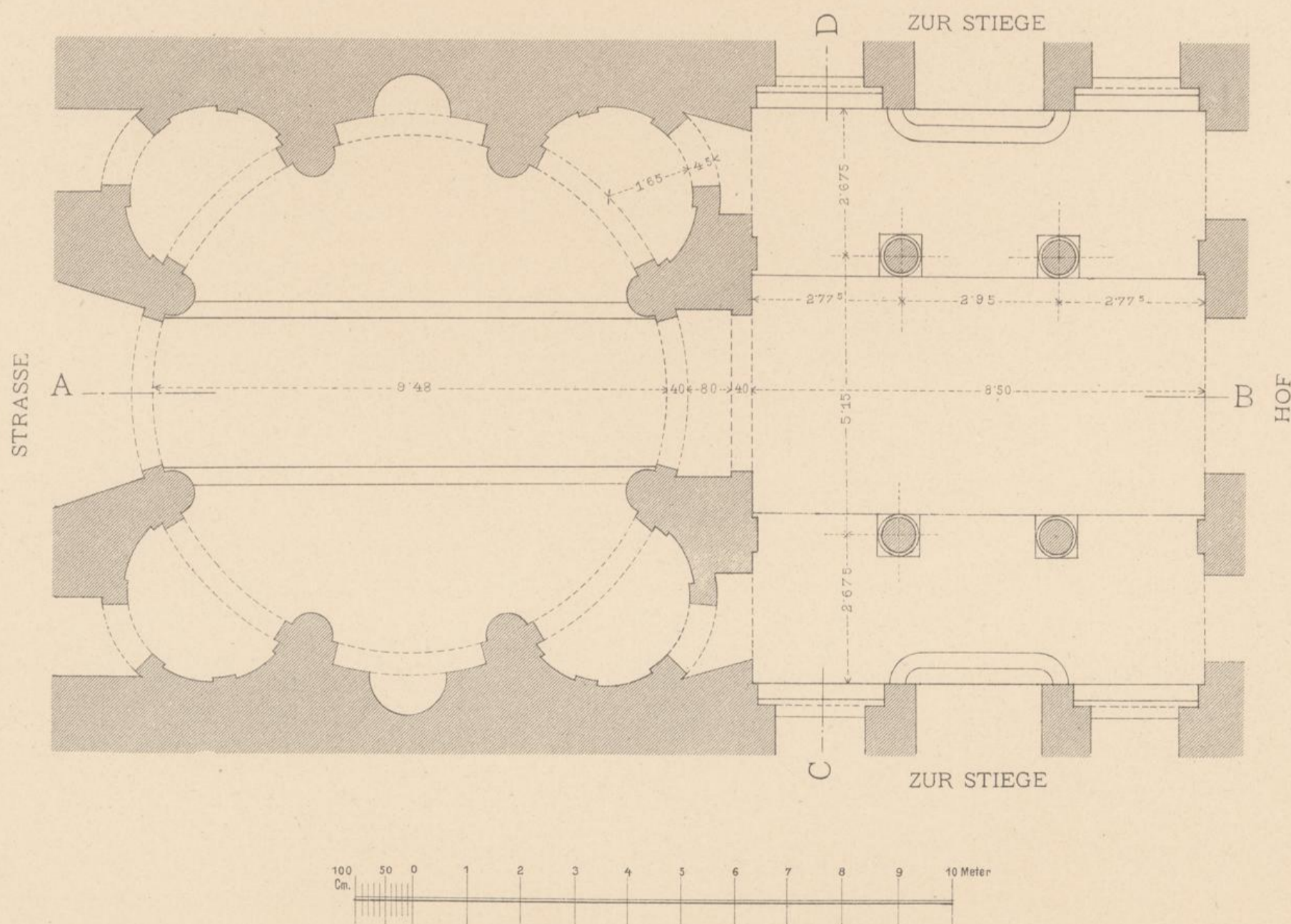
GRUNDRISS
