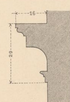
DETAIL DES KLEINEN KÄMPFERS.
