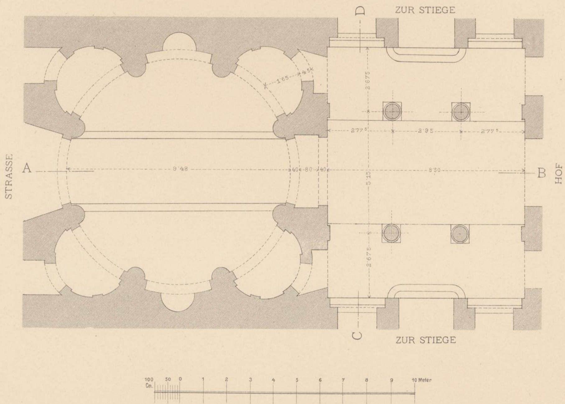
GRUNDRISS
