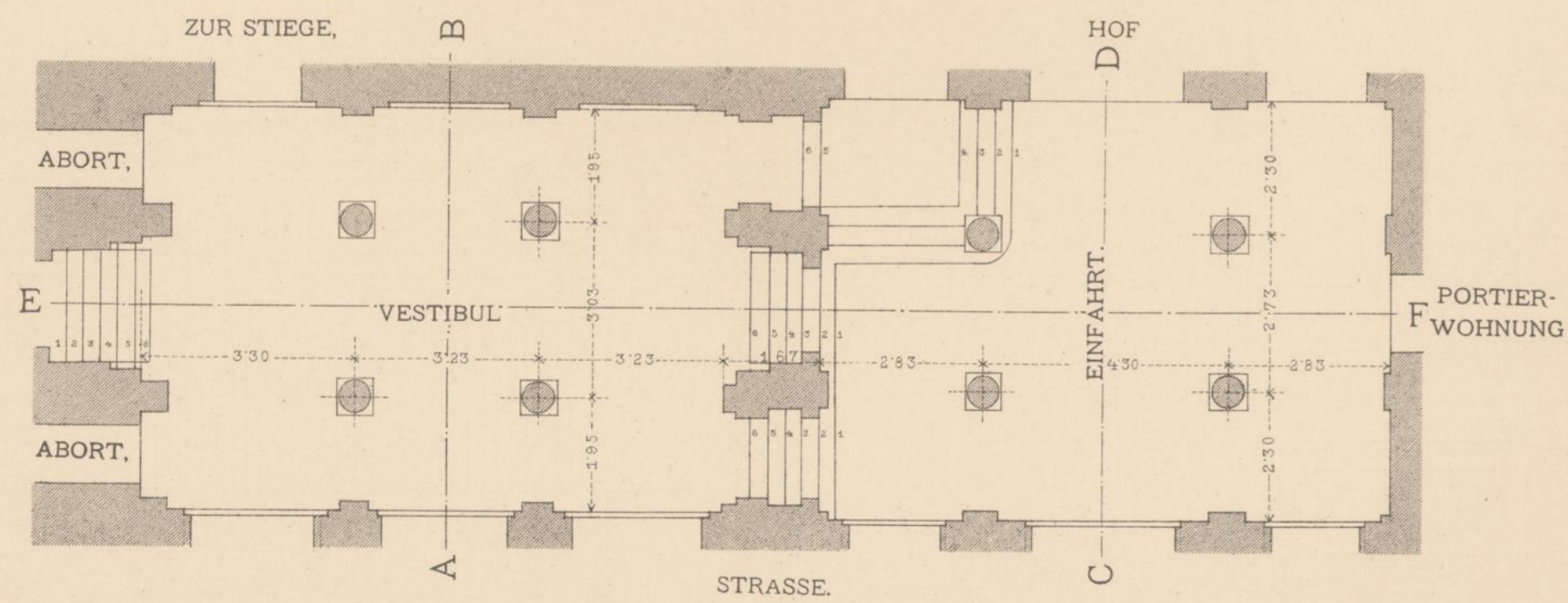
GRUNDRISS
