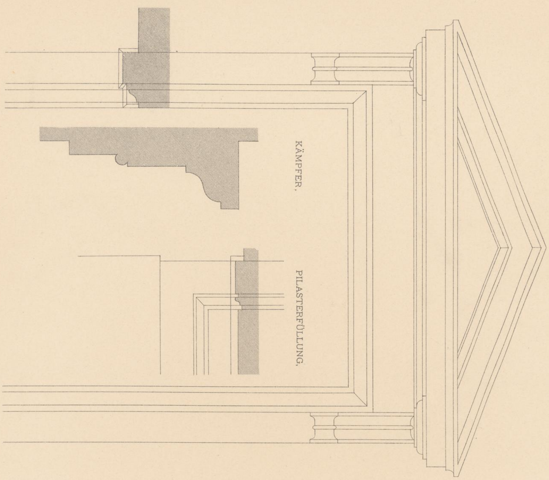
DETAIL DER THÜRE IM VESTIBUL IN 1/10 NAT. GRÖSSE.
