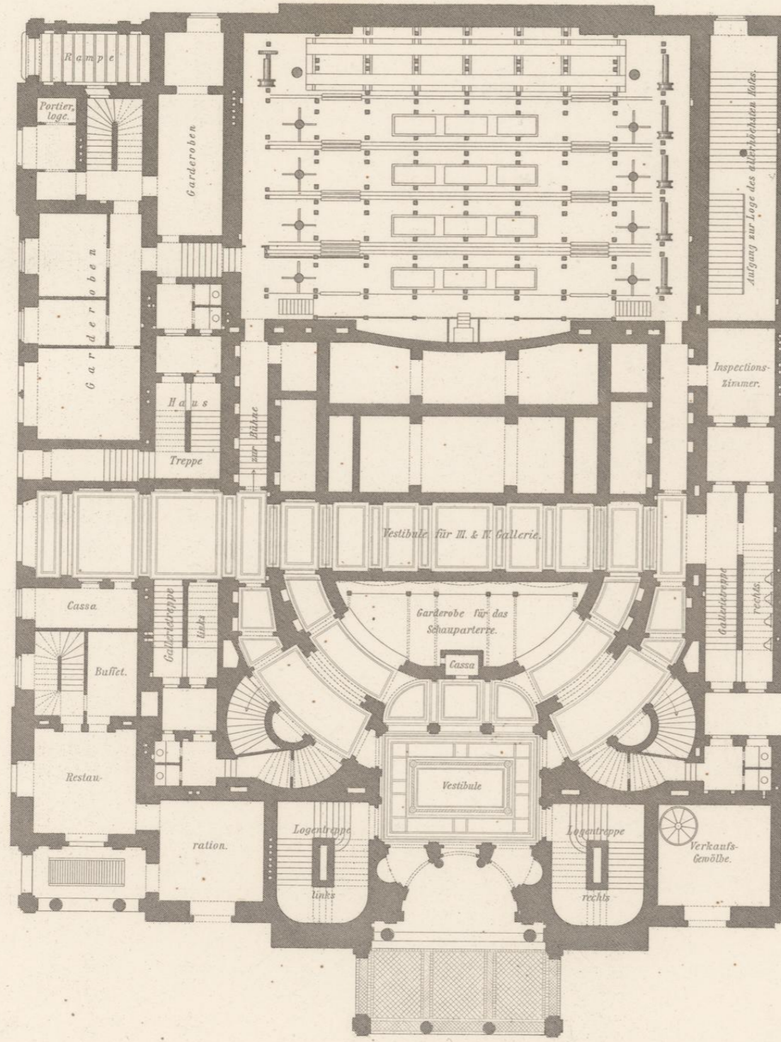
Grundriss des Erdgeschosses zugleich der I. Versenkung.
