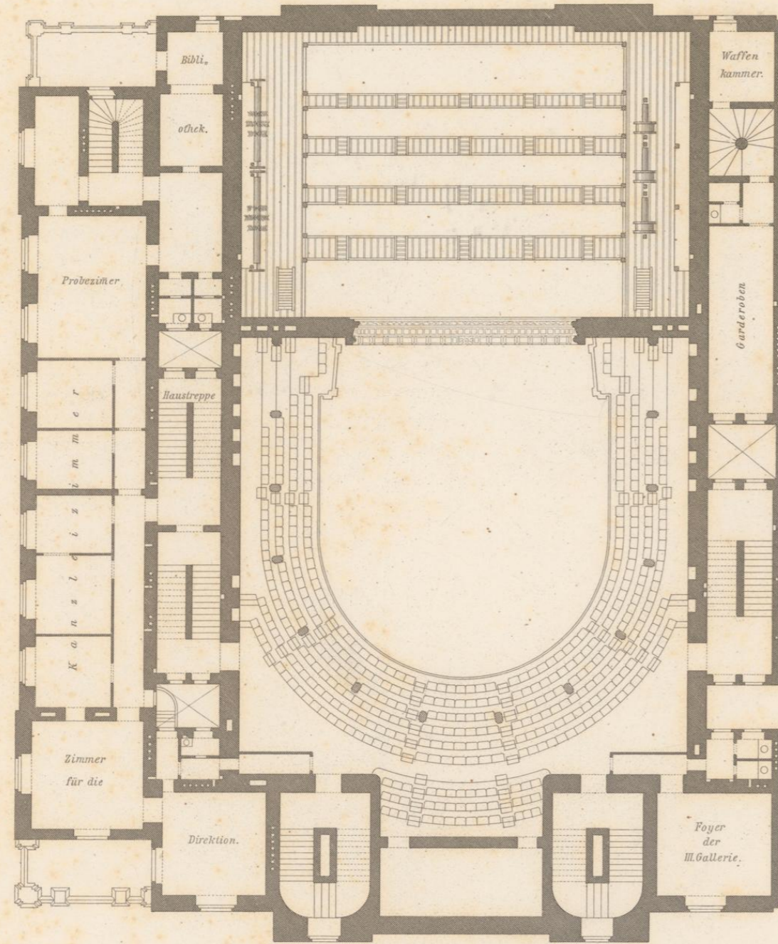
Grundriss des II. Stockes zugleich des III. Ranges.
