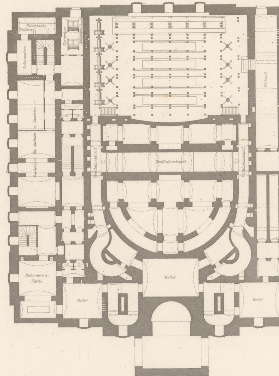
Grundriss des Souterrains zugleich der II. Versenkung.
