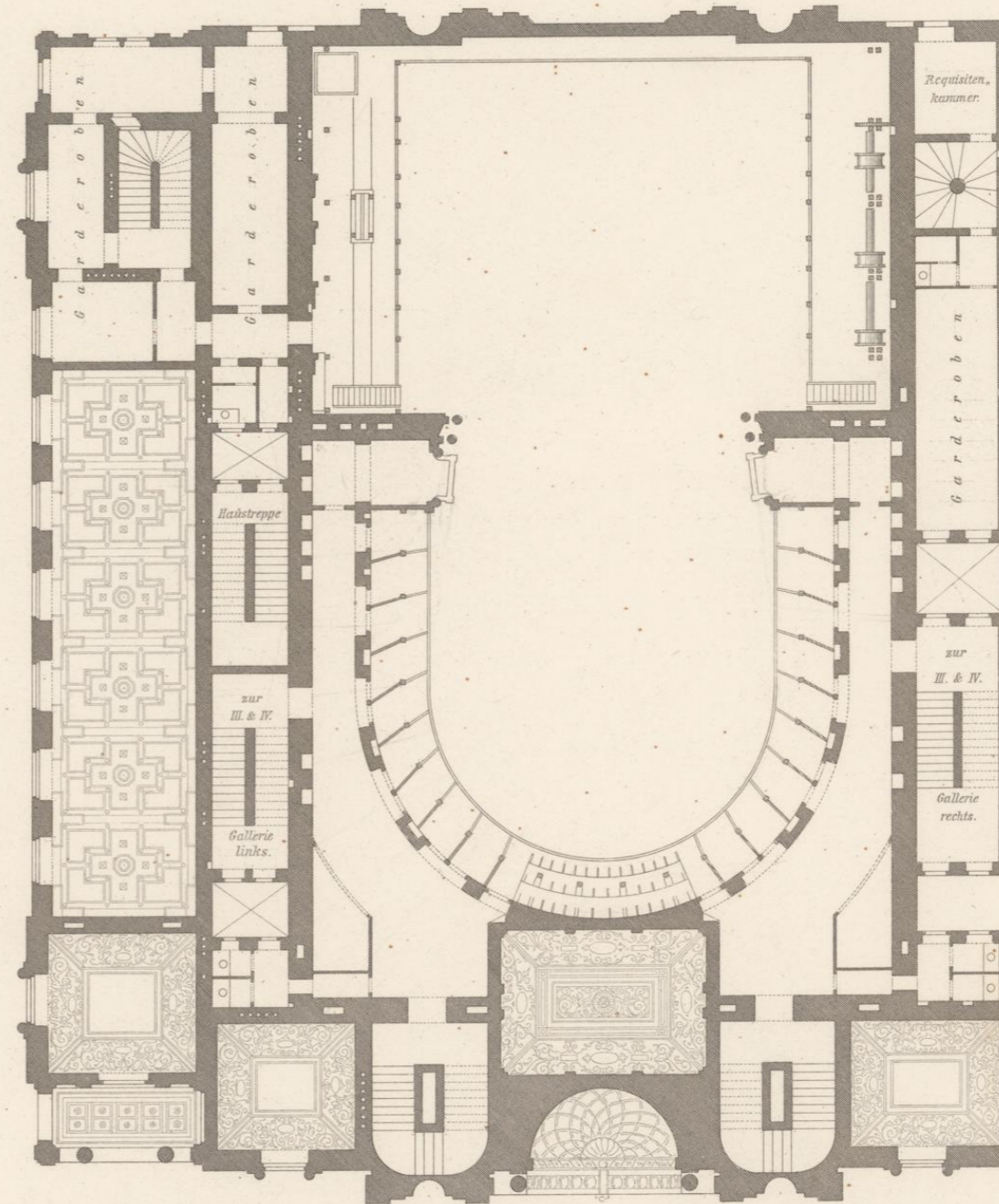
Grundriss der I. Stockuntertheilung zugleich des II. Ranges.
