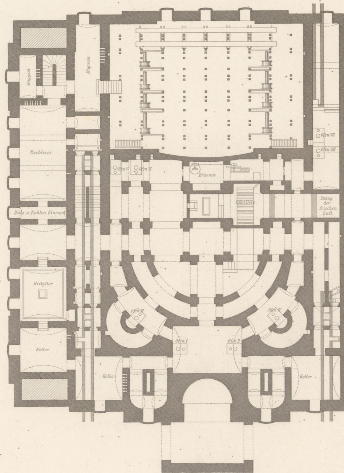
Grundriss des Kellers und der Unterbühne.
