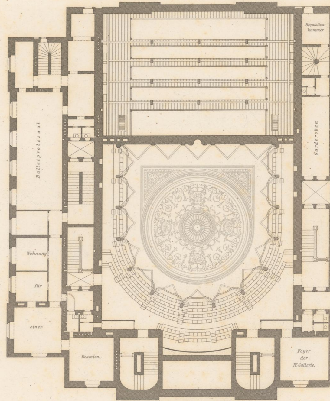
Grundriss des III. Stockes zugleich des IV. Ranges.
