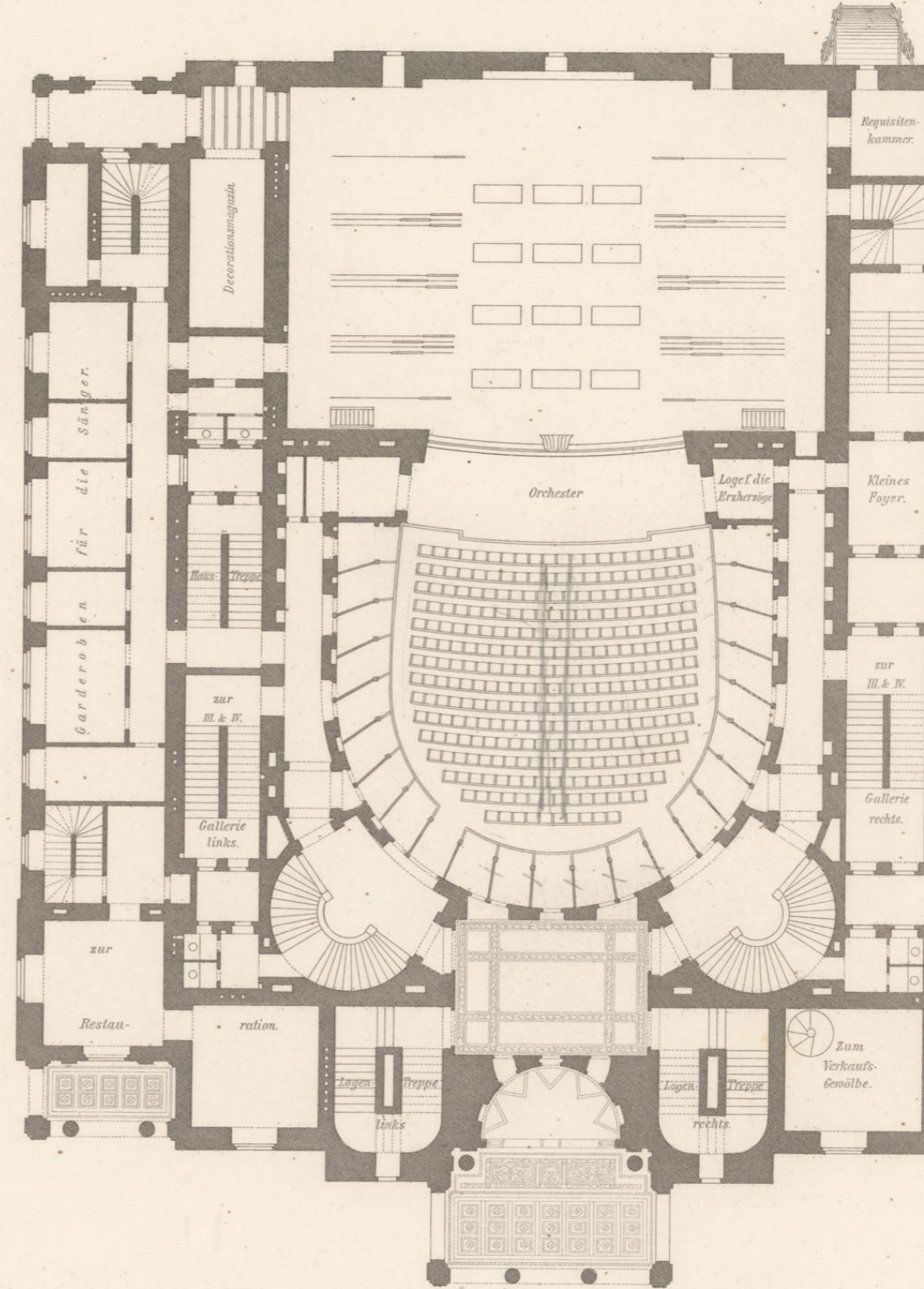
Grundriss des Mezzanins zugleich des Schauparterres.
