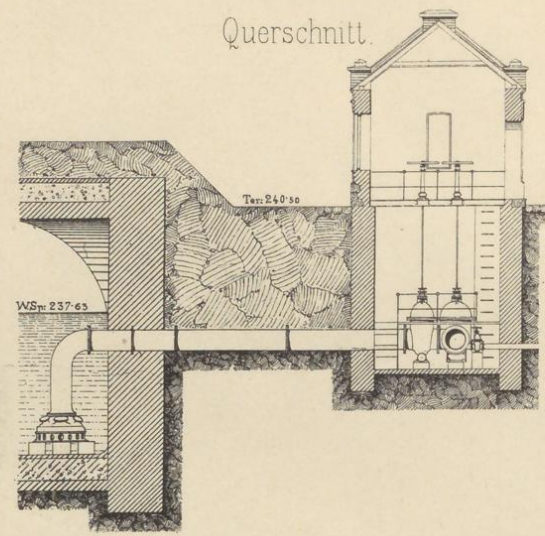
Fig. 2 Schieber-Haus
