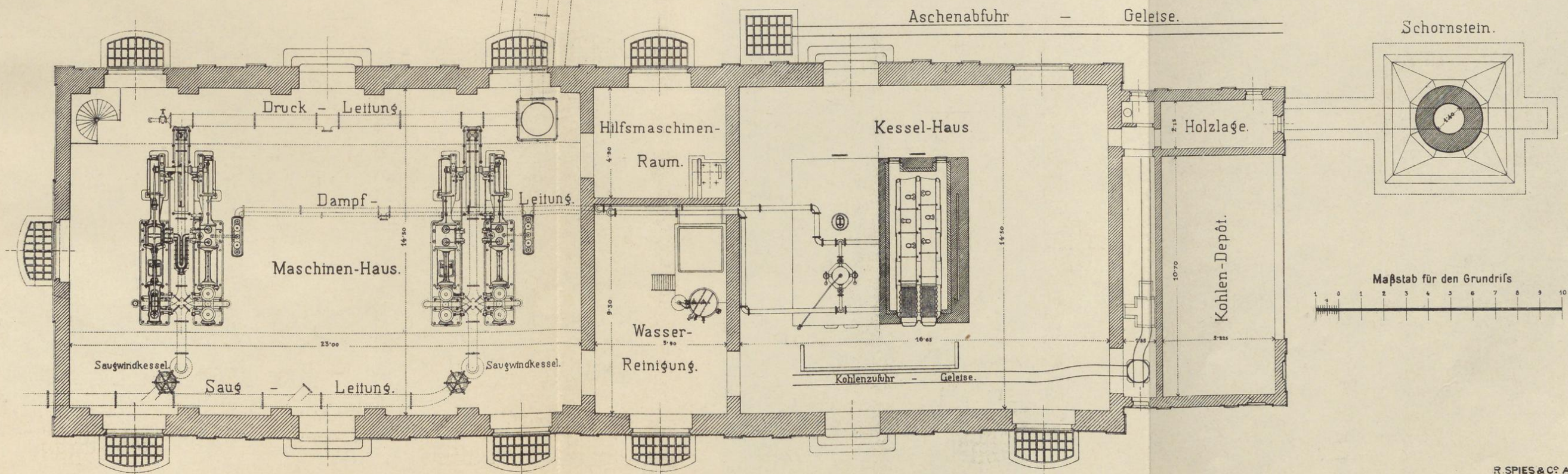
Fig. 3. Grundriss. Parterre.
