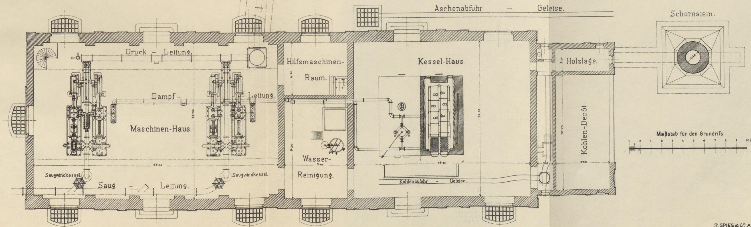
Fig. 3. Grundriss. Parterre.
