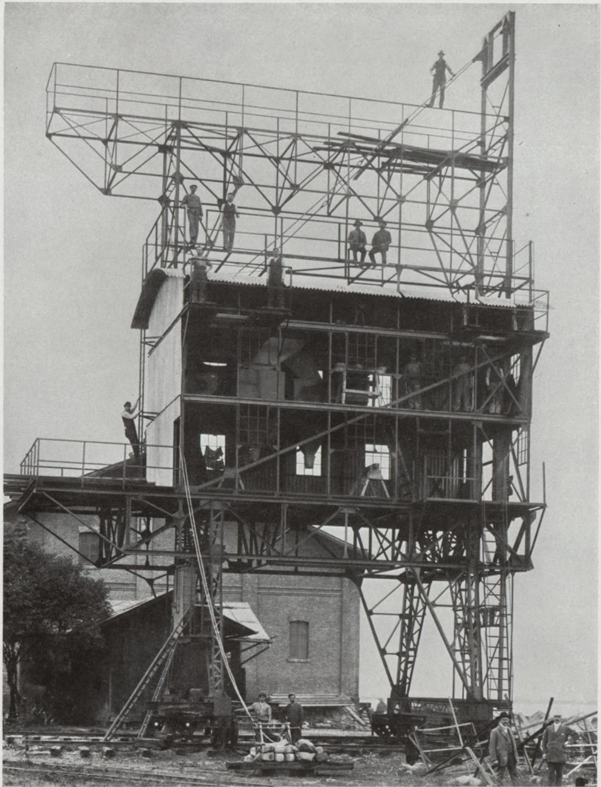
Schiffselevator während der Montierung.
