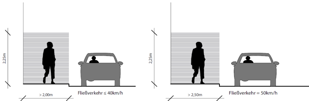
Abbildung 8 Regelbreite Gehsteig, abhängig von Geschwindigkeit auf angrenzender Fahrbahn
